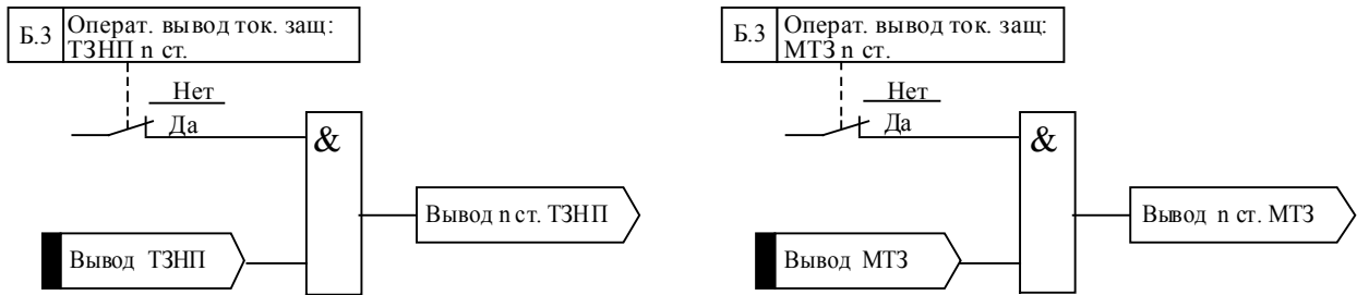
Рисунок 1.3.4 - Функциональная схема формирования сигналов ввода/вывода ступеней ТЗНП и МТЗ
