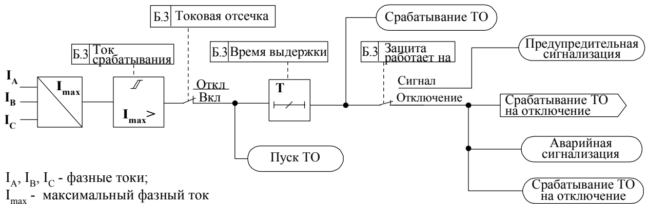
Рисунок 1.3.9 – Функциональная схема токовой отсечки
