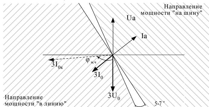
Рисунок 1.3.5 - Диаграмма определения направления мощности нулевой последовательности
