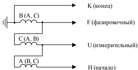
Рисунок 1.3.10 – Схема подключения обмоток ”разомкнутого треугольника” измерительного ТН
