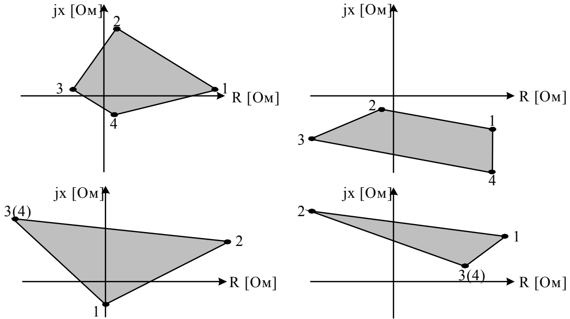
Рисунок 1.3.1 - Характеристики зон срабатывания дистанционной защиты на комплексной плоскости в осях активного и реактивного сопротивления
