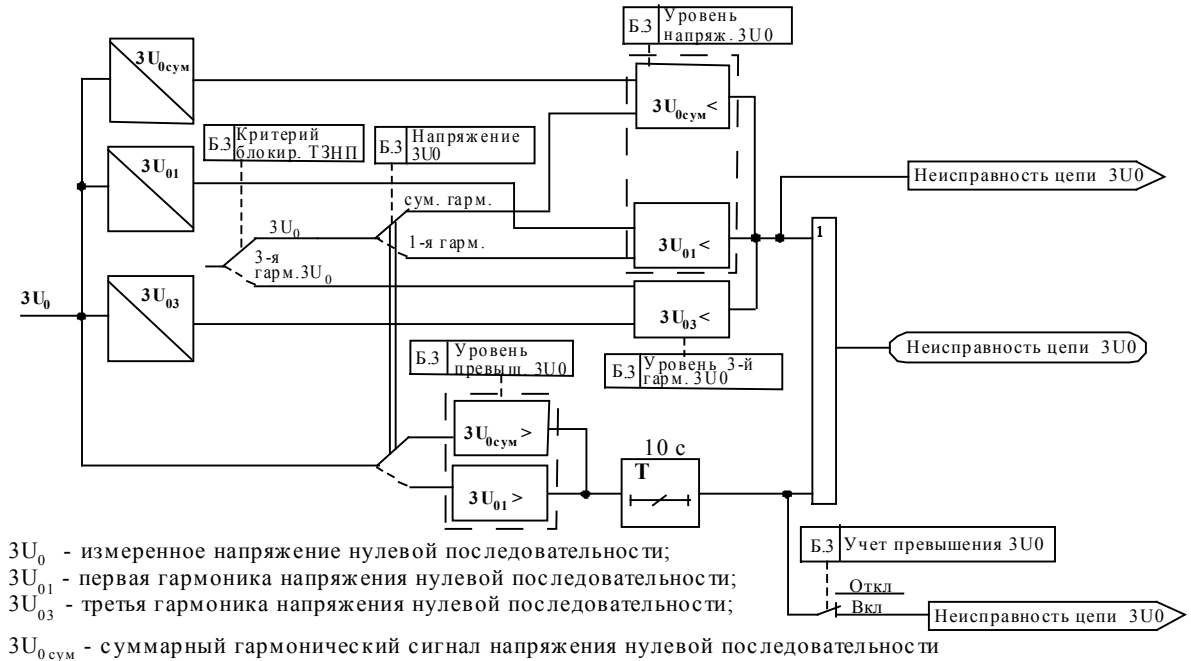
Рисунок 1.3.6 - Функциональная схема формирования сигнала неисправности цепи 3U_0
