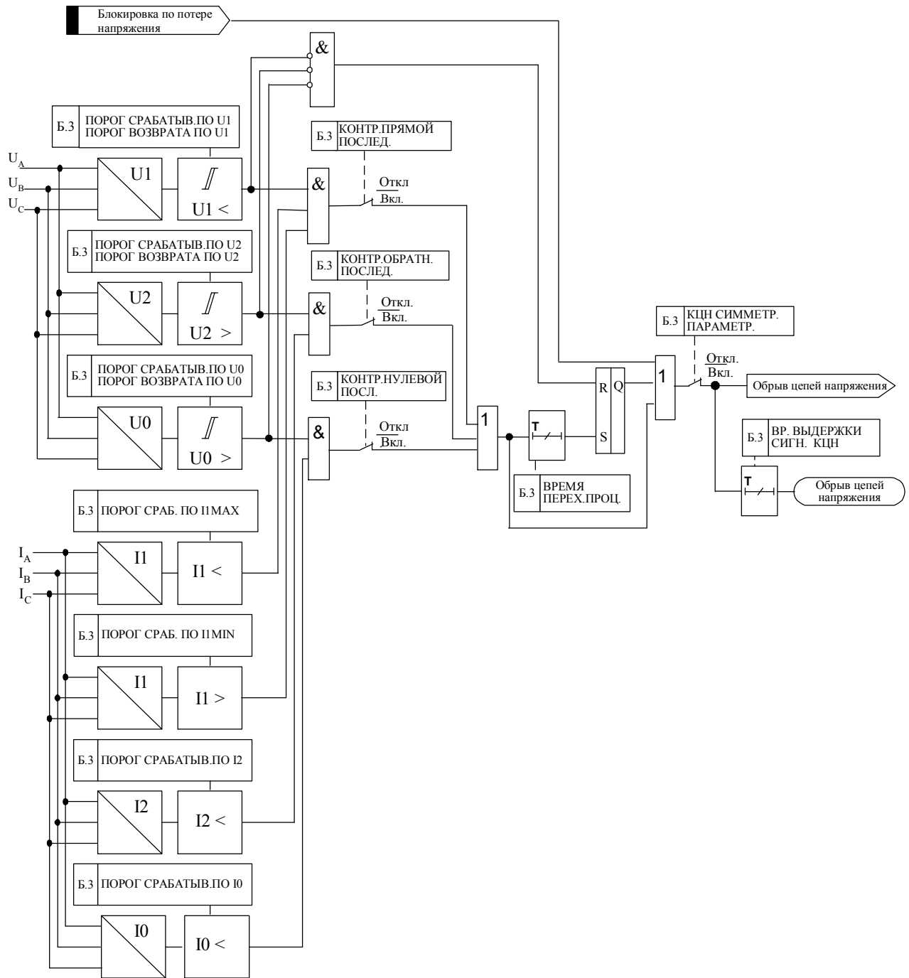
Рисунок 1.3.12 – Функциональная схема контроля цепей напряжения по симметричным составляющим
